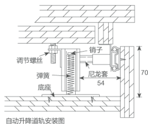
自动升降道轨安装图
