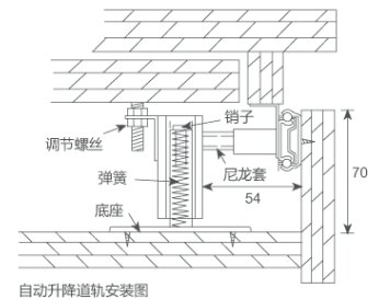
自动升降导轨安装图
